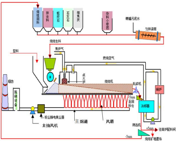
图 1 烧结工艺流程图
