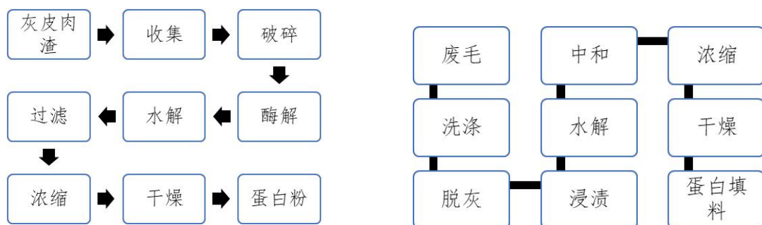
图1 制革灰皮废肉渣清洁化工艺流程
