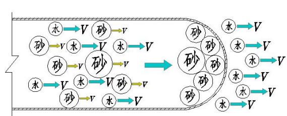
图 2 模袋加压排水固结
